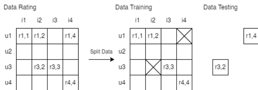
Gambar 3.3. Ilustrasi Pembagian Data
